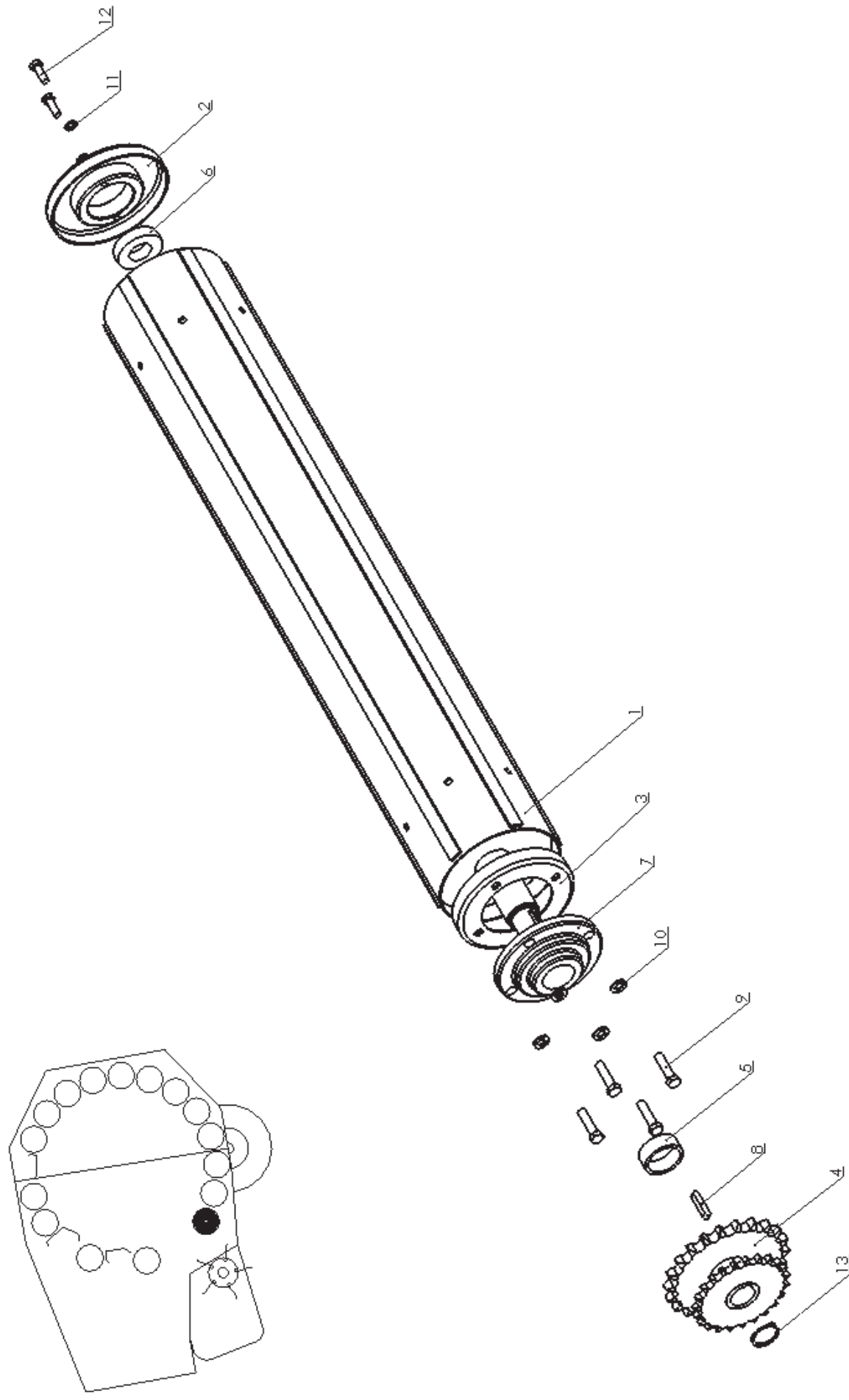
Вал прессующий компл. VI
