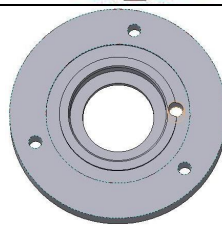
ЛДГ-10М.06.101-01 Крышка Материал: СЧ20. m = 1,54 кг.
